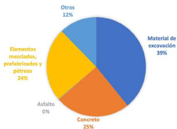
Figura 20. Composición estimada de RCD en México (2011).
